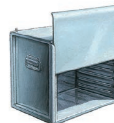
0198 Conteneur traiteur Livré avec 8 grilles pâtisseries 60 x 40 cm. Espace entre les grilles : 6,5 cm. Possibilité de mettre un tiroir chauffant. Ext. : L 66 ; I 43 ; H 71 cm. Int. : L 60 ; I 41 ; H 64 cm. 21 Kg
