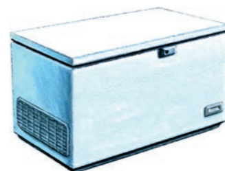
0404 Congélateur 600 L 220 V / 16A monophasé - 290 W. Pouvoir de congélation : 30 Kg / 24 h. Ext. L 165 ; P 81 ; H 89 cm. 75 Kg
