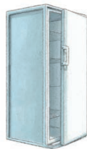
0327 Réfrigérateur 250 litres : 220 V / 16A 180 W. Ext. : L 60 ; I 56 ; H 137 cm. 45 Kg
