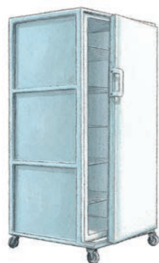
0684 Réfrigérateur 500 litres : 220 V / 16A 150 W. Ext. : L 75 ; I 70 ; H 151 cm. 75 Kg. Livré avec 5 grilles 68 x 52 cm. Ext. : L 80 ; I 80 ; H 180 cm.
