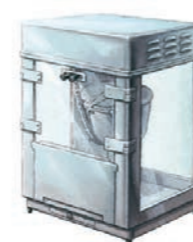
0379 Machine à pop-corn 220 V / 16A monophasé - 1,6 kW. Chauffe contrôlée par thermostat. Livrée avec une pelle à pop-corn Ext. : L 47 ; l 43 ; H 78 cm. 44 Kg En complément : cornets à pop-corn page 91
